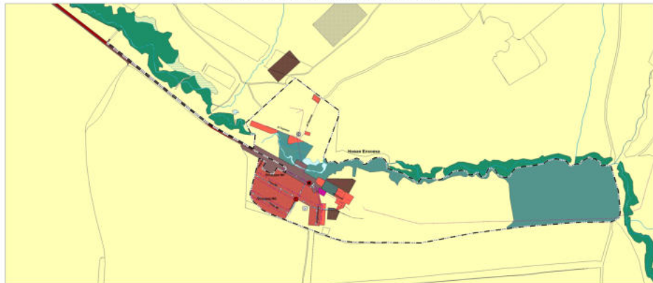
Карта планируемого размещения объектов инженерной инфраструктуры местного значения с. Нероновка муниципального района Сергиевский Самарской области
